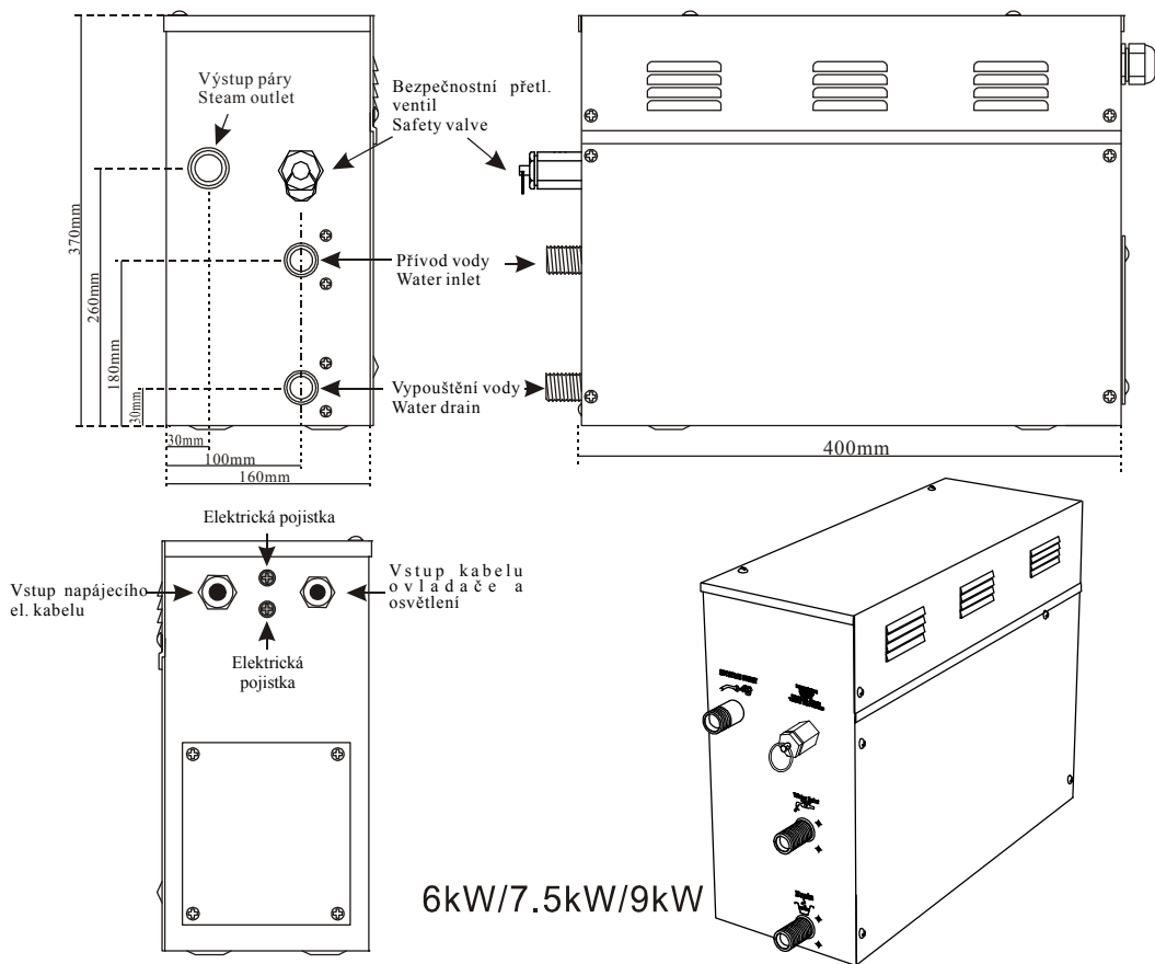
Obr. 3 Nákres parního generátoru 3-9kW.
